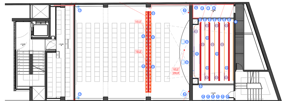
PLANTA PRIMERA
