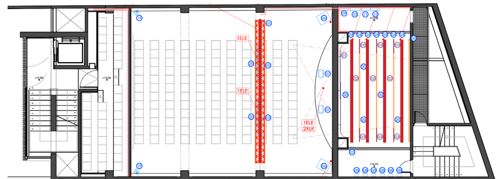
PLANTA PRIMERA
